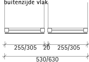
Tweedelig acryl, aan de buitenzijde vlak
