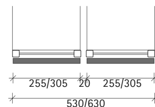
Tweedelig hout, vlak aan de buitenkant
