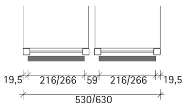
Tweedelige houtsoort, binnenin gelegen
