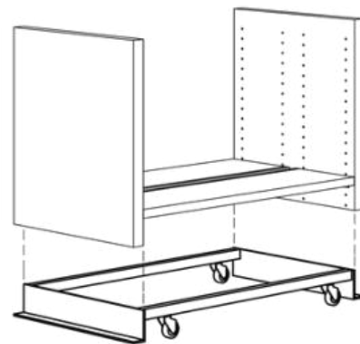
Trolley voor dubbele planken
