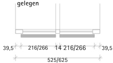
Tweedelige houtsoort, intern gelegen
